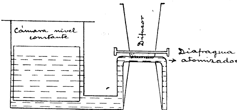
Corte esquemático del nuevo carburador nacional «Simplex K-63»
